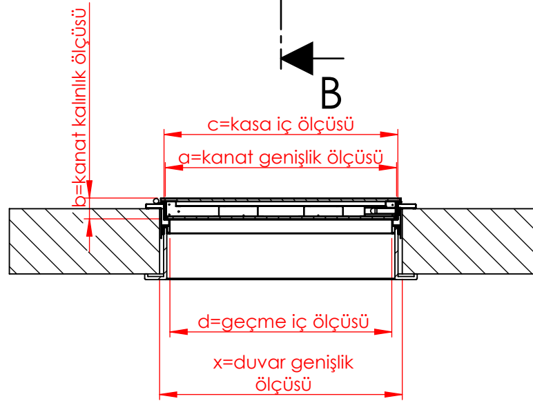
KESİT A-A ÖLÇEK 1 : 20
