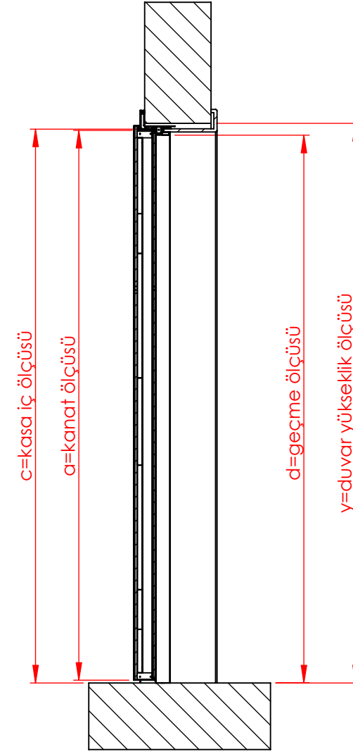
KESİT B-B ÖLÇEK 1 : 20
