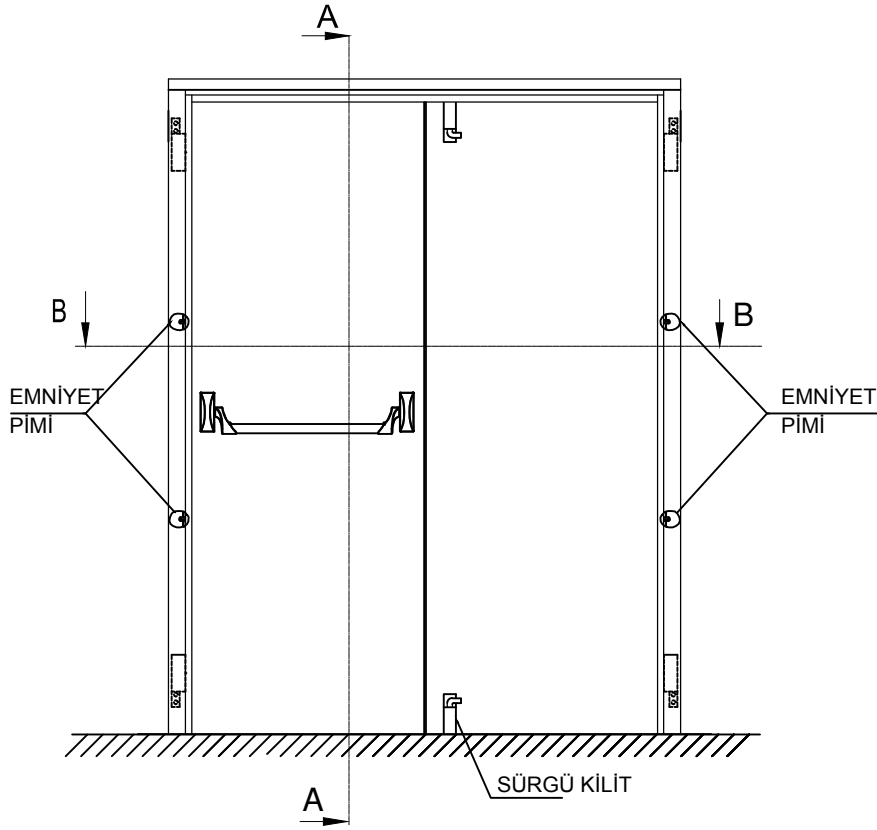
A-A KESİTİ
